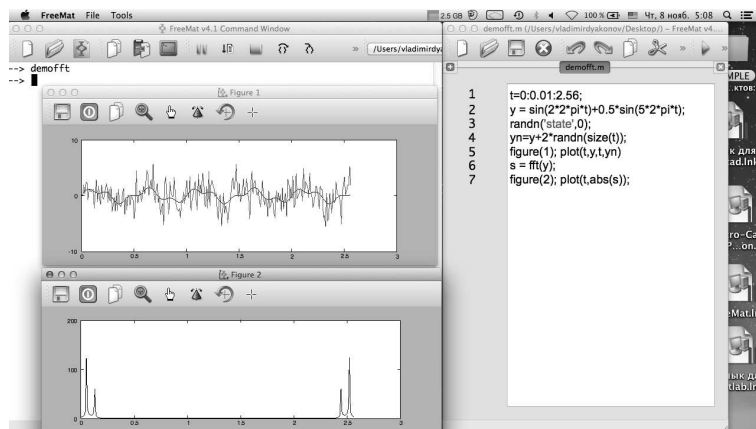
Рис. 8: Пример создания файла demoftt.m и исполнения команды demoftt .
