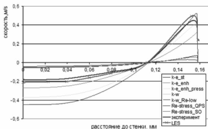
Рис. 3: Распределения скорости от оси симметрии двухмерной модели до стенки, полученные при использовании различных моделей турбулентности.
