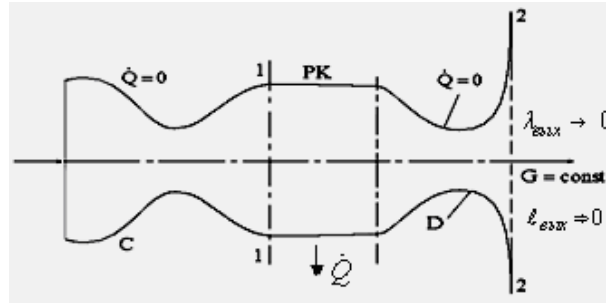
Рис. 1. Принципиальная схема поточной газовой системы ( L_{tech} = 0 ), \lambda_{вых} – коэффициент скорости потока на выходе из системы, \ell_{вых} – момент количества движения на выходе из системы, C – сверхзвуковое сопло, PK – пространство поточной системы, где отводится (или доводится) энергия \bar{Q} , D – диффузор.
