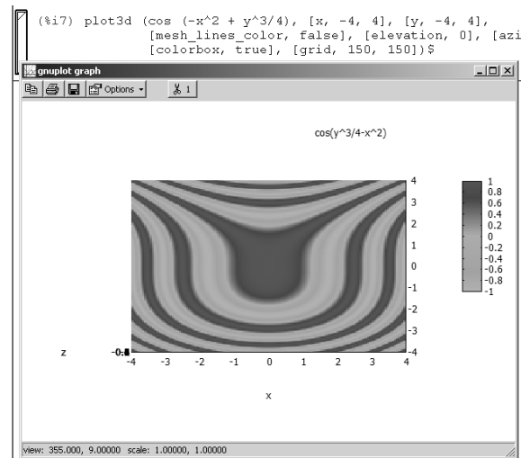
Рис. 51: Контурный график поверхности с высотой, представляемой цветом.
