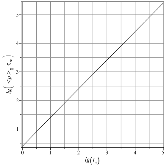
Рис.7. Зависимость безразмерного временного параметра \tau_\infty \langle \tilde{p} \rangle_0 от временной космологической постоянной; всюду N_0 = 100; N = 10, p_0 = 10; \sigma_0 — снизу вверх: 0.01; 0.1; 0.2; 0.5.
