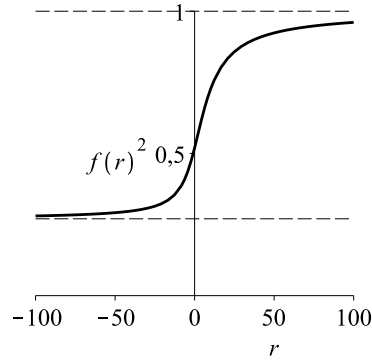
Рис. 3: Пример поведения функции f^2 при M = 2, Q_e = 1, Q_d = 10 .
