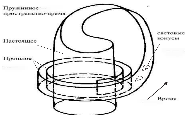
Рис.1. Пространство-время, свернутое в пружину в объемлющем пятимерном Гиперпространстве.
