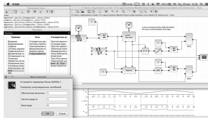
Рис. 25: Применение блока IF.
