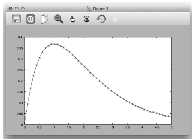
Рис. 7: Пример приближения полиномом 6-степени функции с падающим участком.
