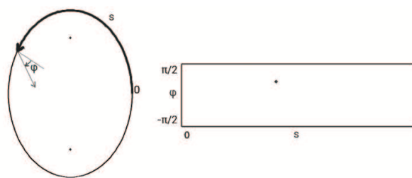
Рис. 4: К построению фазового пространства эллиптического бильярда.
