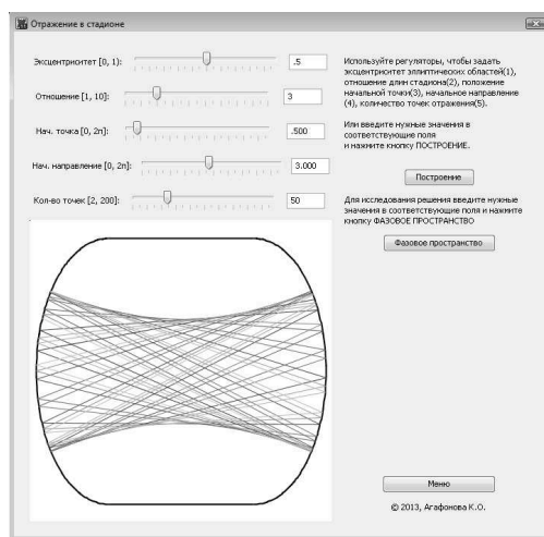
Рис. 7: Вид макета для моделирования и визуализации бильярда на столе в в форме стадиона.
