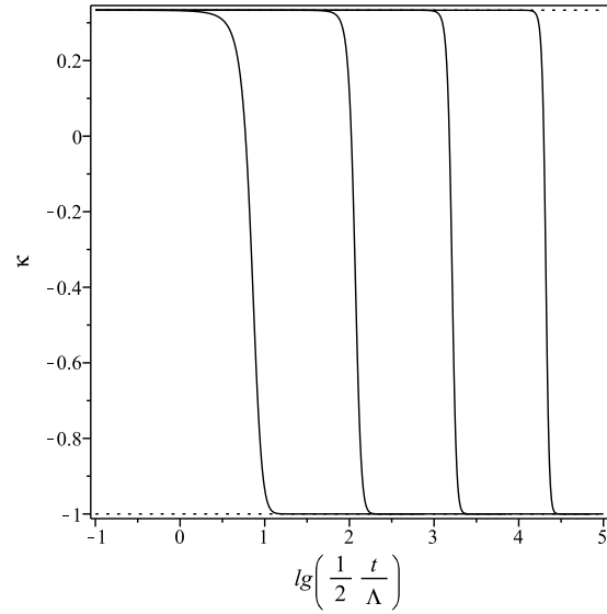
Рис.5. Эволюция эффективного коэффициента баротропы \kappa(t) относительно точного решения (141) в зависимости от космологической постоянной \Lambda слева – направо: \Lambda = 1 , \Lambda = 10 , \Lambda = 100 , \Lambda = 1000 .
