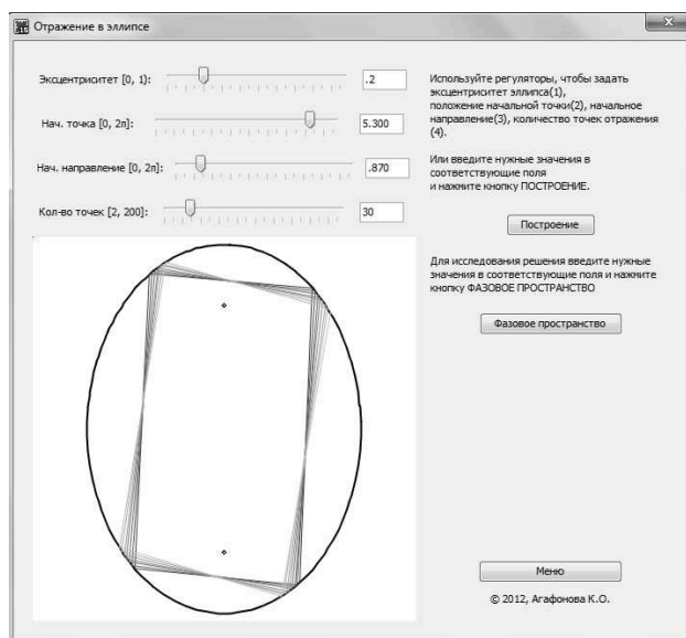
Рис. 2: Вид маплета для моделирования и визуализации бильярда на столе эллиптической формы.
